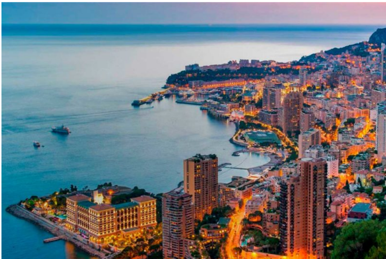
Monte Carlo
